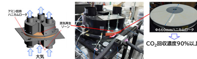
蒸気再生ハニカムロータリーDAC（1,000m 3 /h規模）実験
