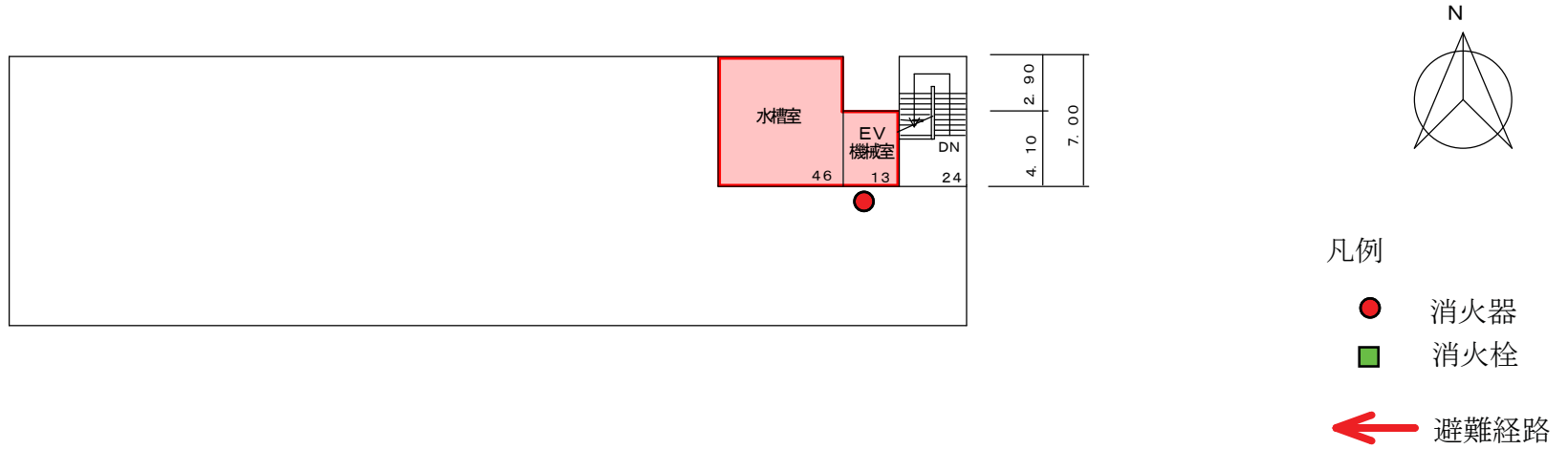
屋階平面図
