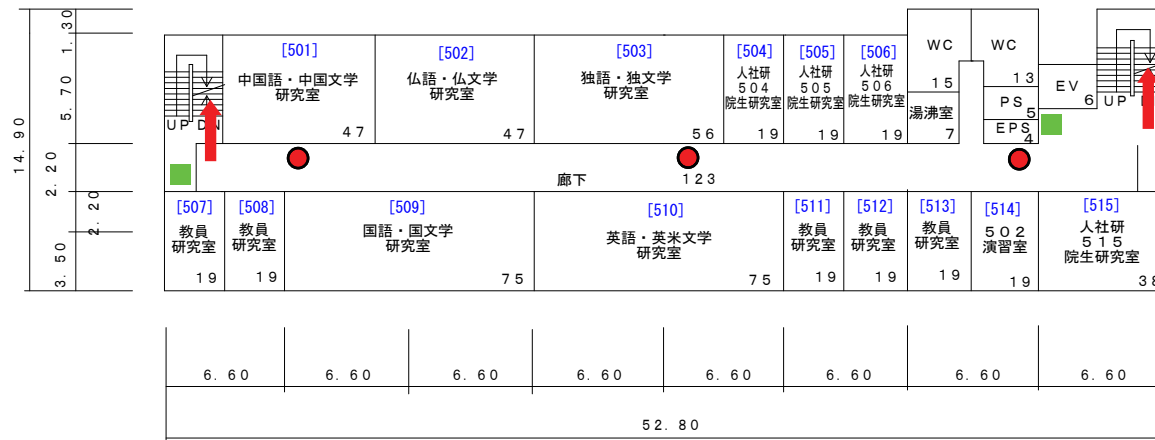
5 階平面図
