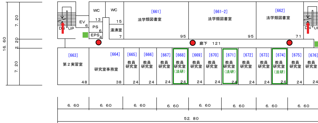
6 階平面図
