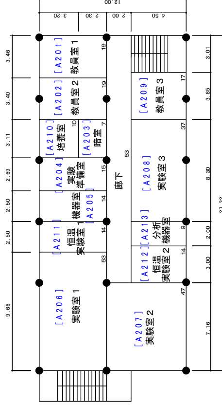
2階平面図 328㎡
