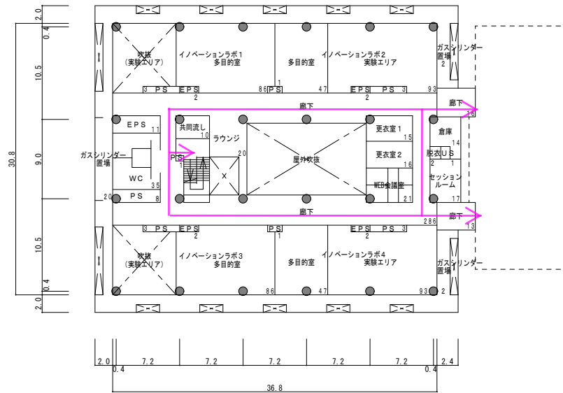
5階平面図
