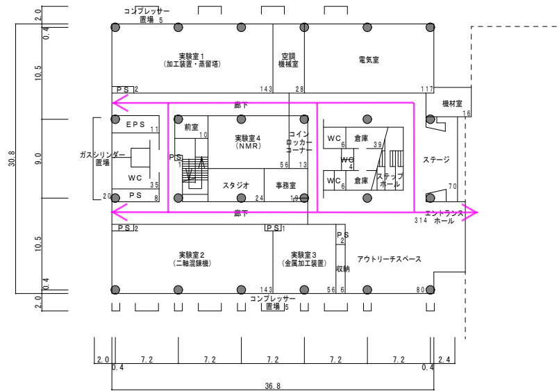
1階平面図
