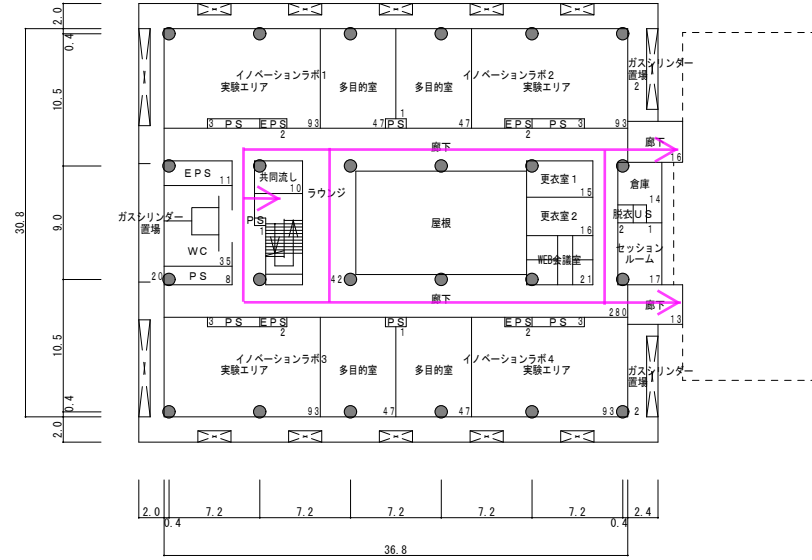
4階平面図
