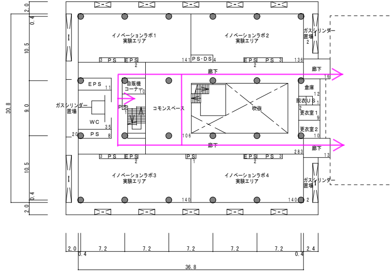
3階平面図
