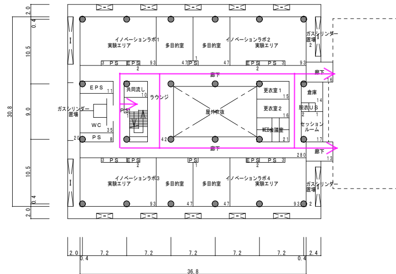
6階平面図
