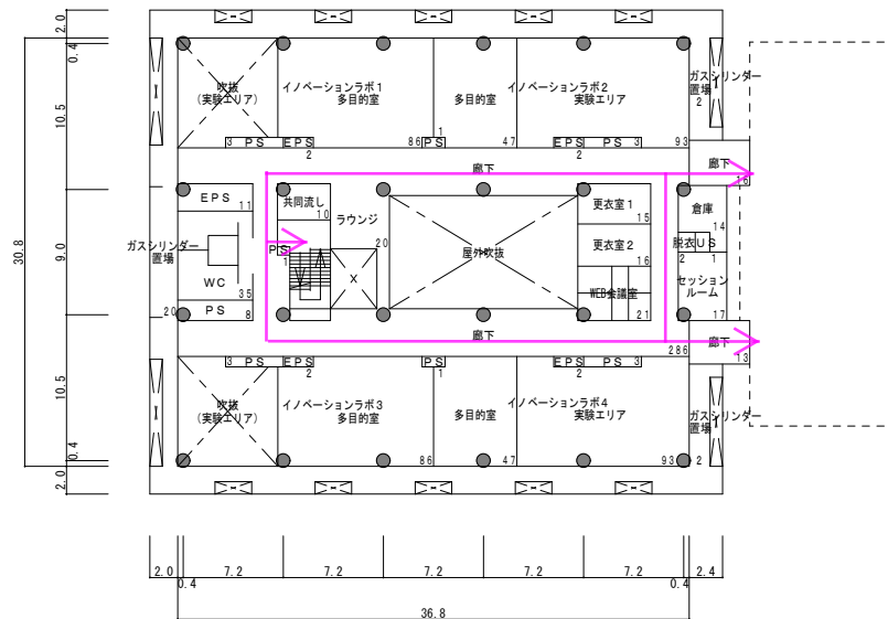
5階平面図
