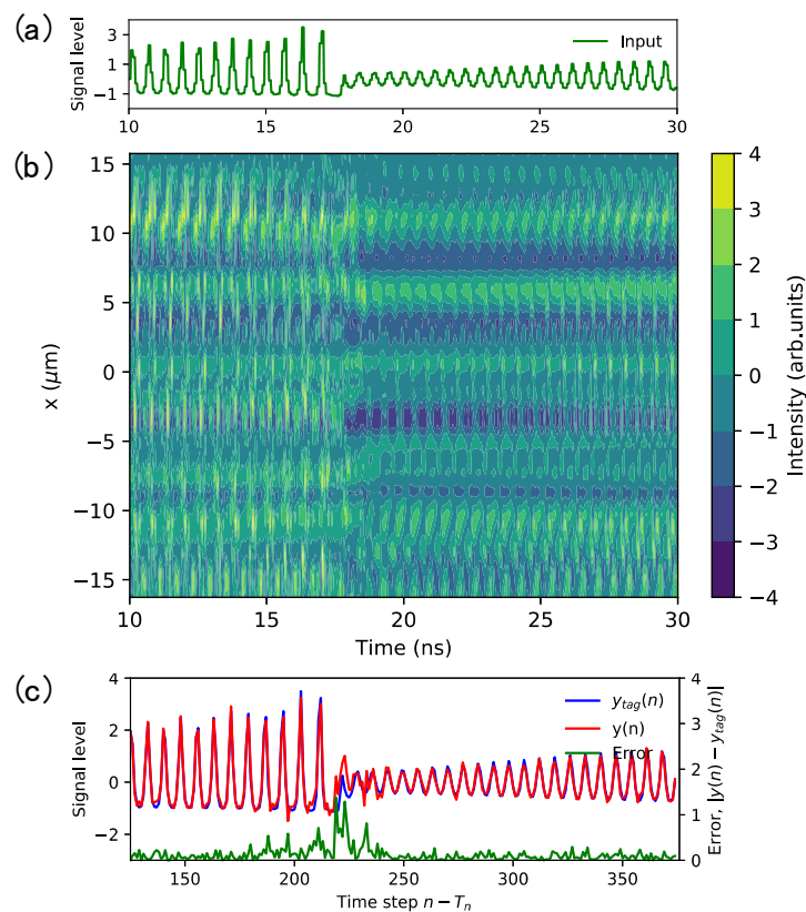
図 3. カオス的な複雑信号の 1 ステップ先を予測した結果
