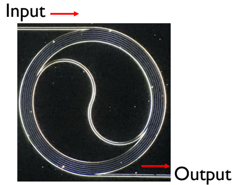
図 2. 本研究で作製した光リザーバ計算回路チップ
