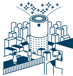
エアロゾルを精密に計測する研究
