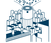
エアゾルを精密に計測する研究
