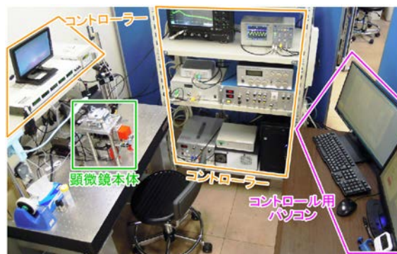
実験に使用した高速 AFM の写真
