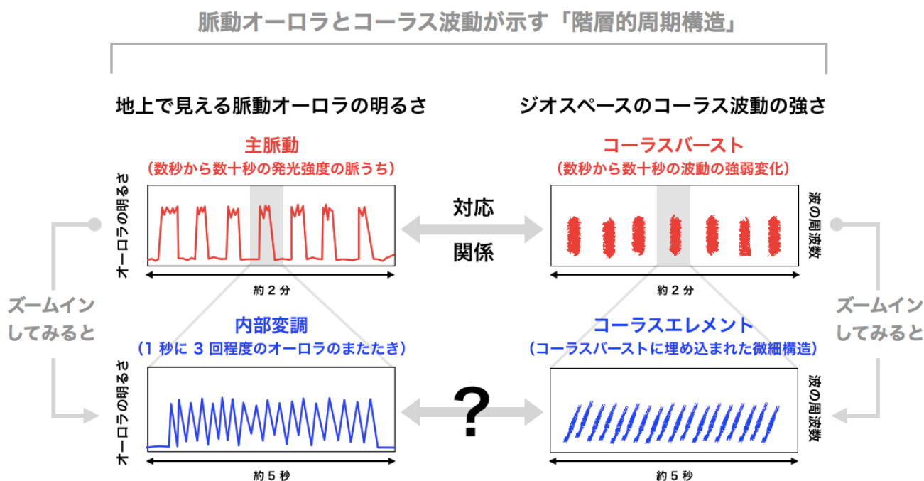
図 2: (左) 赤線は数秒から数十秒のペースで明滅する脈動オーロラの「主脈動」を表す。主脈動の明るくなっている時間（山の部分）をズームインすると、青線で描いたような 1 秒間に 3 回程度明滅する「またたき（内部変調）」が存在することが知られている。(右) 赤線は、コーラス波動が集団的に発生する様子（コーラスバースト）を示す。このコーラス波動の時間変化が脈動オーロラ的主脈動をコントロールしていることが、近年の科学衛星「あらせ」による観測によって示されている。このコーラスバーストをズームインすると、「コーラスエレメント」と呼ばれるコーラス波動の「さえずり」が見られることが知られている。コーラスエレメントと脈動オーロラの内部変調（またたき）の間に関連があることが予想されていたが、宇宙と地上での同時観測による実証がなされていなかった。
