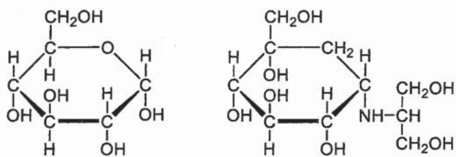
図1 \alpha -グルコース(左)とボグリボース(右)の構造式
