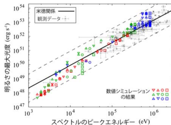
図 米徳関係と数値シミュレーションの結果の比較
