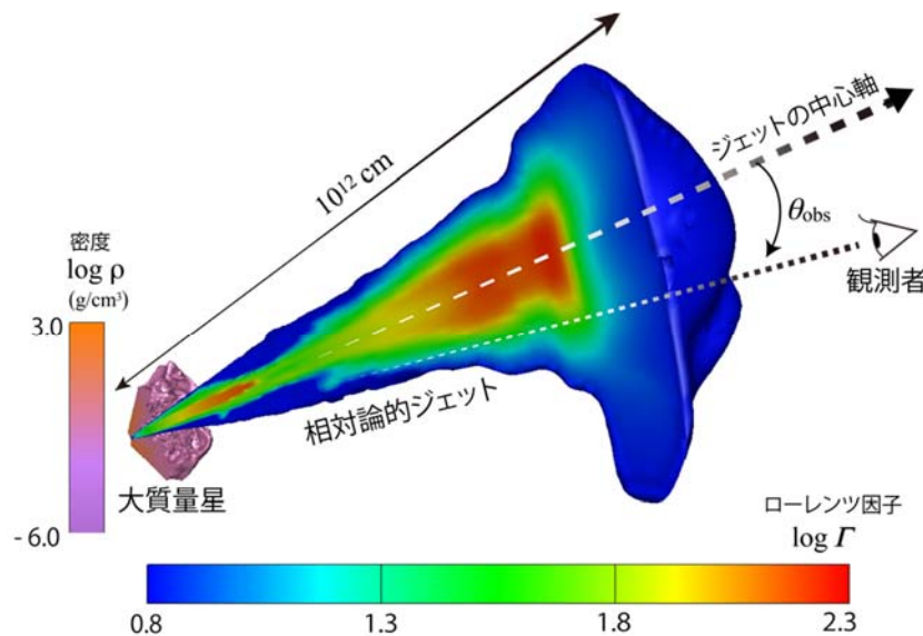
図1 大質量星を突き破るジェットの相対論的流体シミュレーション
