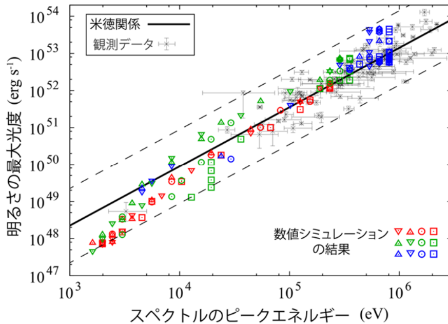
図2 米徳関係と数値シミュレーションの比較
