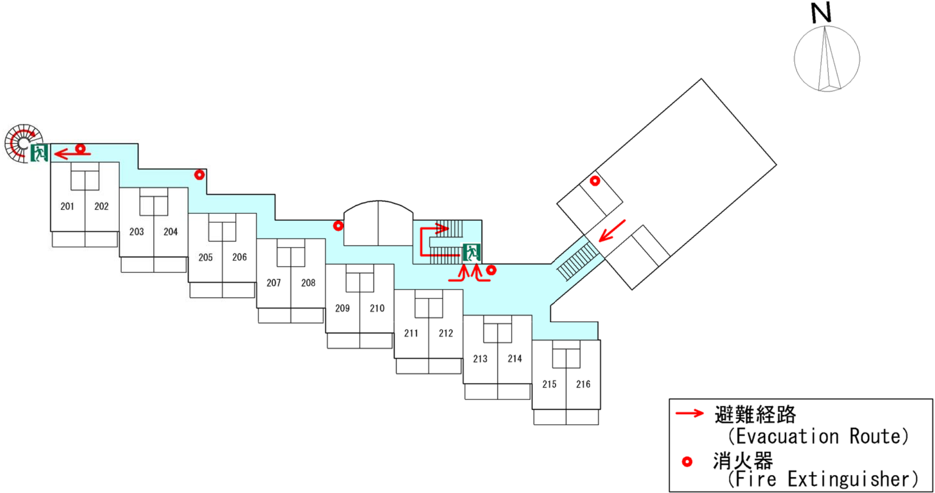
国際交流会館 2階平面図 Layout of 2nd Floor, International House
