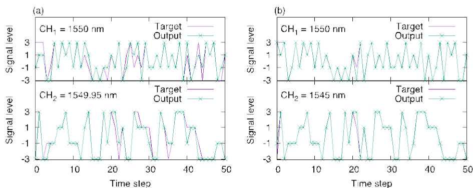
図 4. 2つの独立の非線形・ノイズ通信路から得られた別々の受信信号を1つのスペckル生成器（マルチモードファイバ）を用いて同時に復元推定した結果。通常、1つの計算デバイスに2つの信号を入力すれば、(a)で示すように、信号が干渉して推定に失敗する。一方、本提案のデバイスでは、光波長多重化技法の援用により、(b)のように高精度に信号復元が可能となる。
